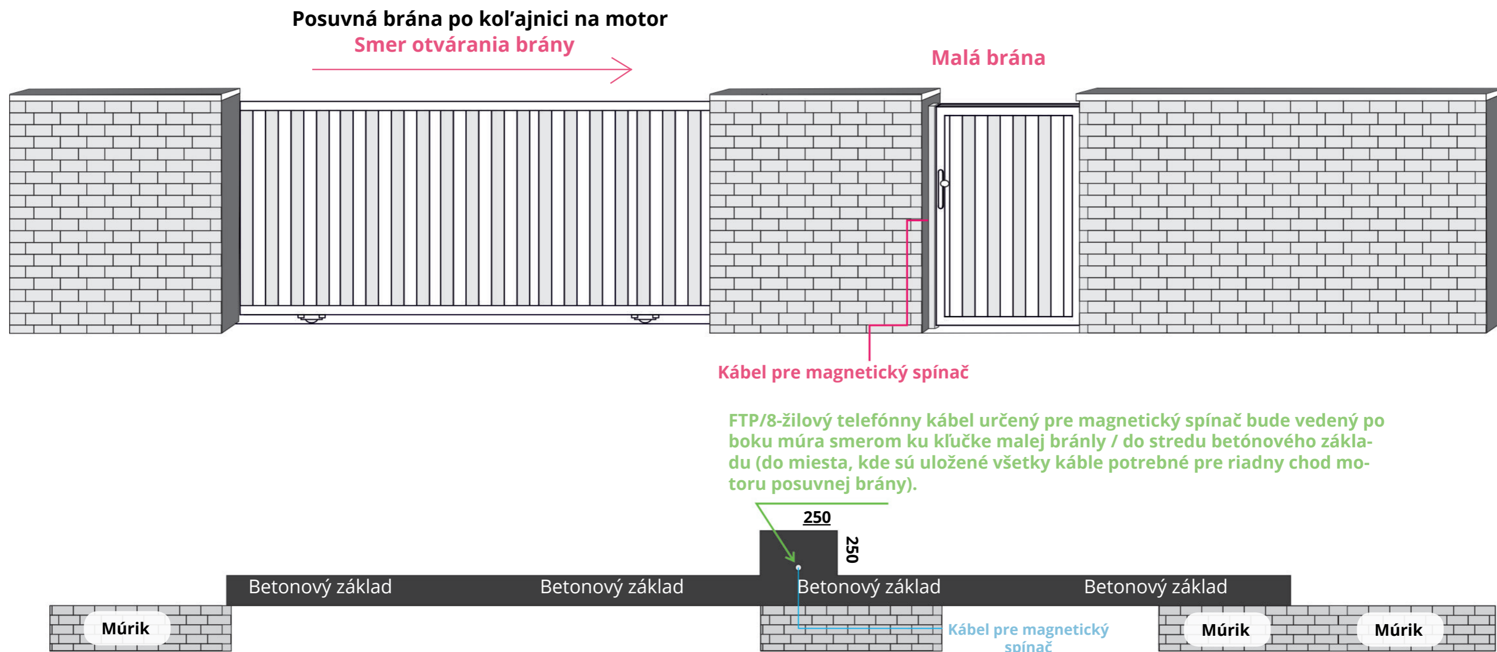
Pohľad zhora na múrik a betónový základ pre posuvnú bránu
